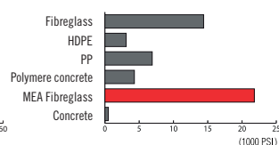
Tensile strength
